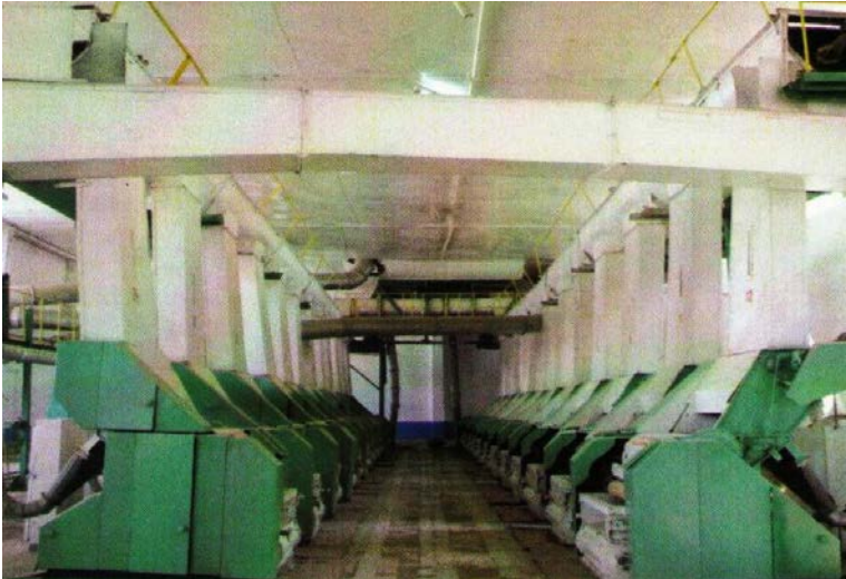
Şəkil 39. Pambıqtəmizləmə zavodlarında ДВ -1М markalı fırlanan silindrlı (barabanlı) cin maşınlar sistemi
