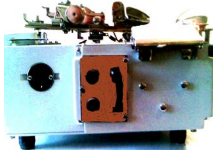
Şəkil 54. MПPШ -1 cihazının ümumi görünüşü
