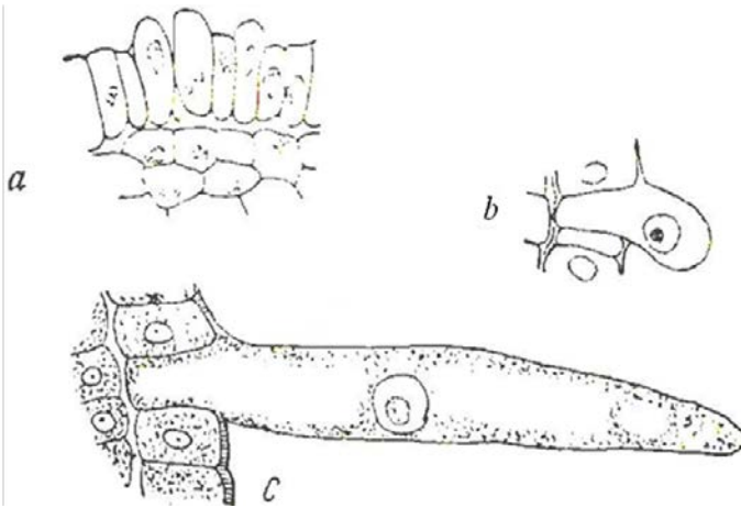
Şəkil 8. Pambıq lifinin inkişafı: a – epidermis hüceyrələrinin çiçəkləmə günündə vəziyyəti, b - çiçəkləmənin səhəri stüündəki. c - çiçəkləmədən 2 stün sonrakı vəziyyəti
