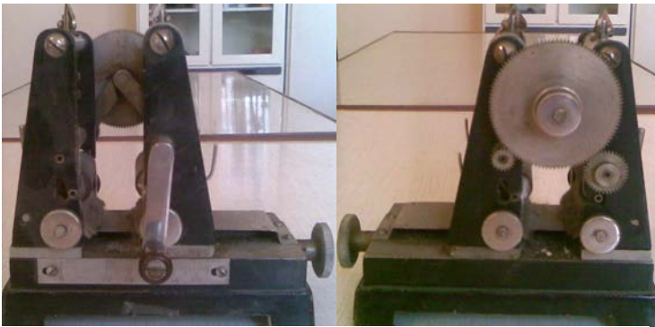
Şəkil 45. Laboratoriya üçün kiçik Jukov cihazı (hər iki tərəfdən görünüşü)
